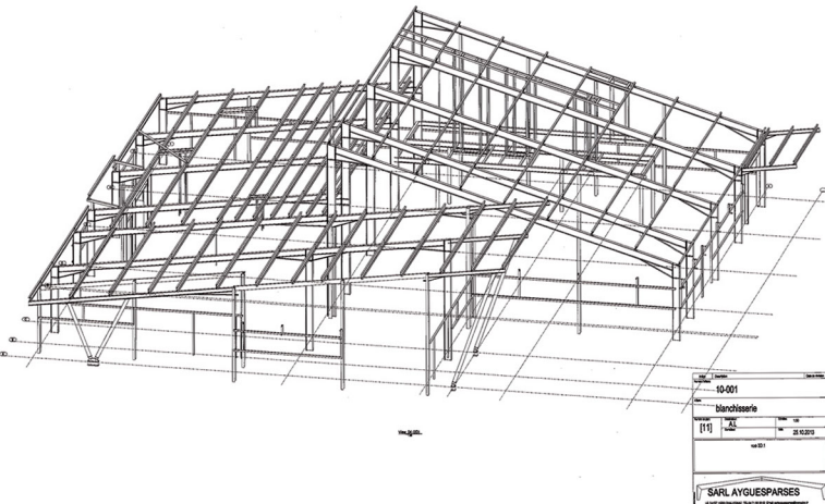
Plan 3D, blanchisserie, Bort les orgues (19)
